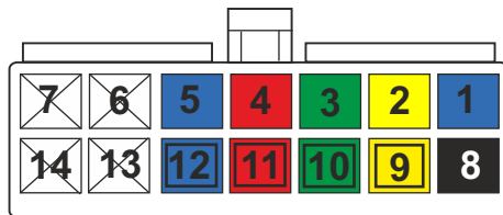
Vista Trasera -Salida de Cables
